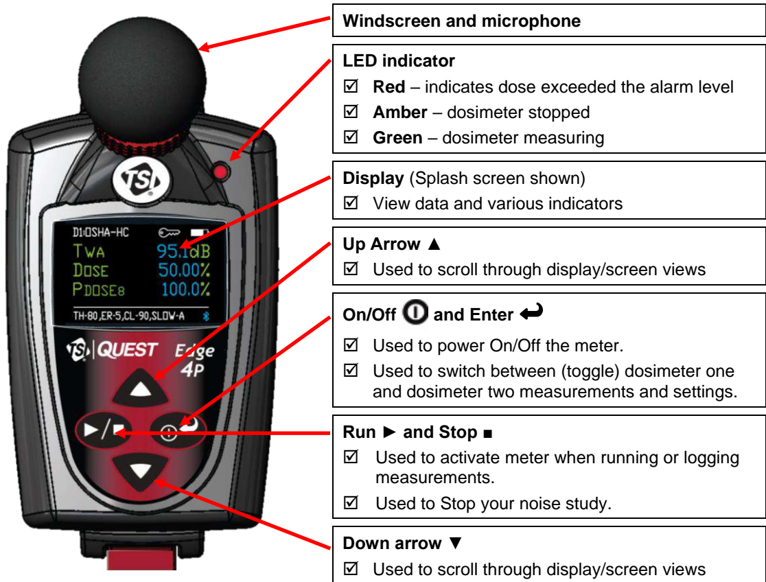
Figure 2-4 Edge Keypad
