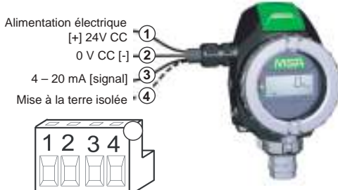
Connexion à 3 fils – PrimaX P
