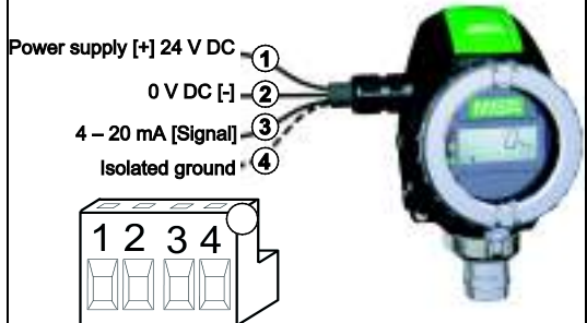
3 сымды қосылым - PrimaX P
