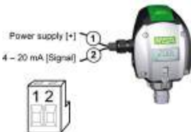
2-жична връзка – PrimaX I
