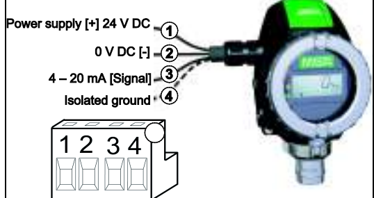
Conexiune cu 3 fire - PrimaX P
