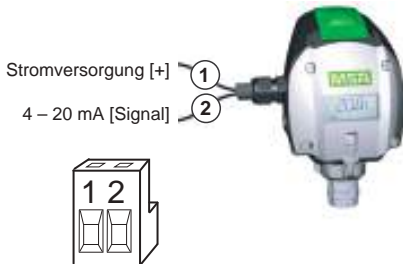
2-adrige Verbindung – PrimaX I
