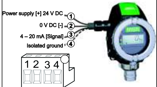
3-жична връзка – PrimaX P
